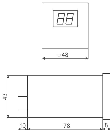
Maßbild KM ZAD 24/2
