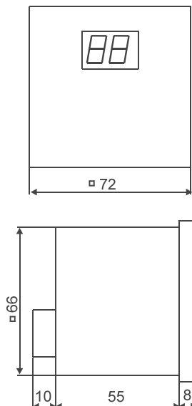
Maßbild KM ZAD 220, KM ZAD 24
