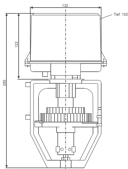
Maßbild
